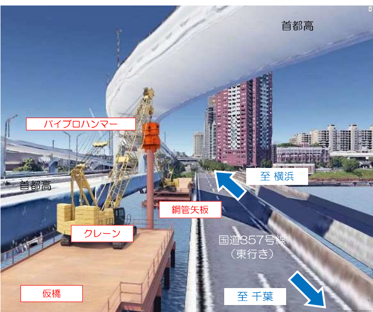
鋼管矢板打設状況イメージ図
