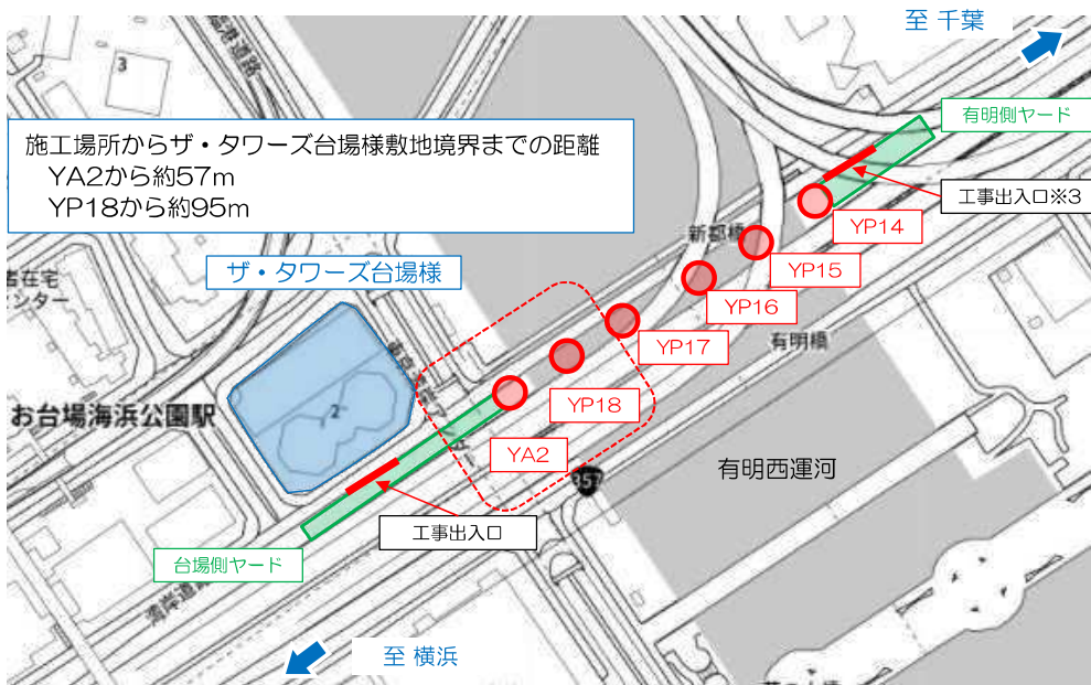
平面図
